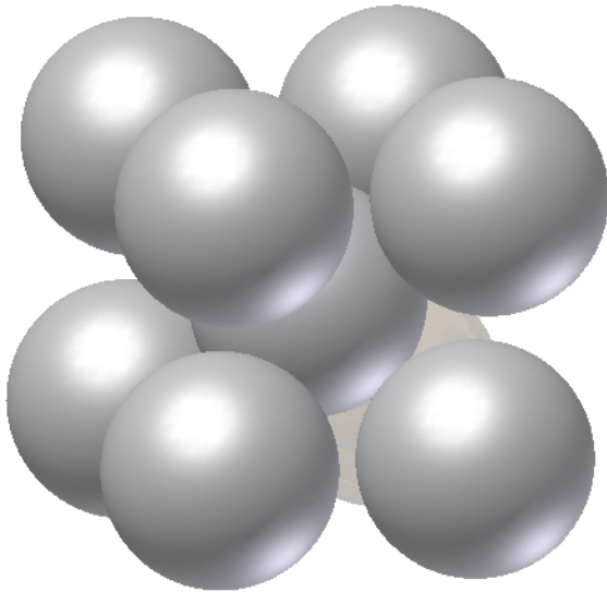
Kubisch-raumzentriert (krz)
