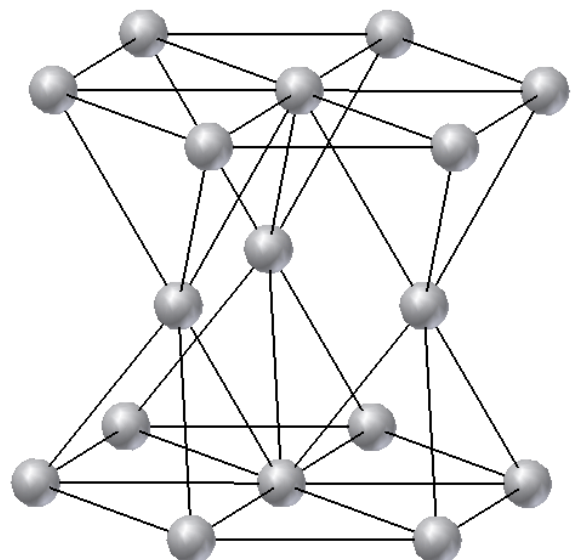
hexagonal (hex) bzw. hexagonal dichtest gepackt (hdp)
