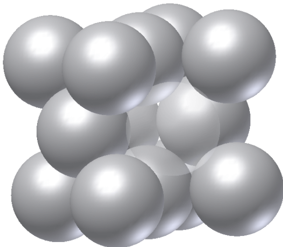
Kubisch-flächenzentriert (kfz)
