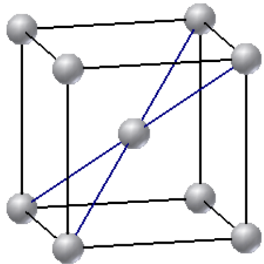
Kubisch-raumzentriert (krz)
