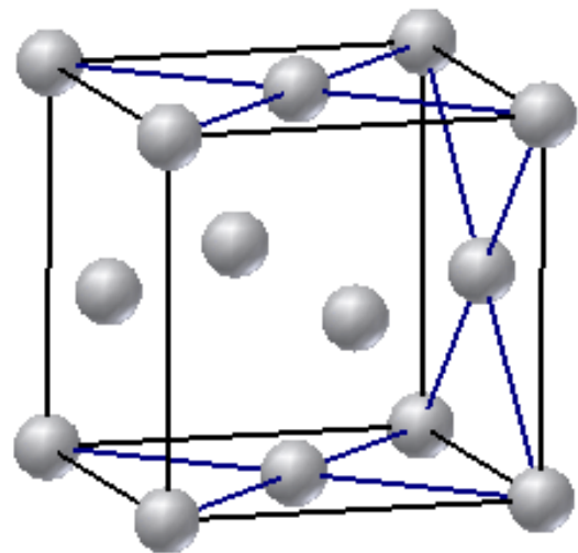
Kubisch-flächenzentriert (kfz)
